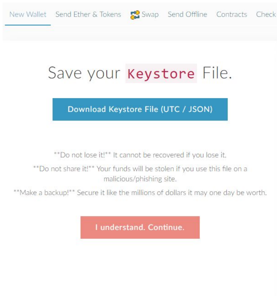
Рис. 3. Инструкции
