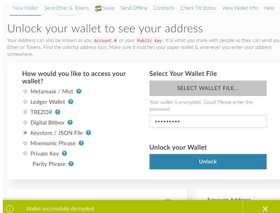
Рис. 6. Разблокировка
