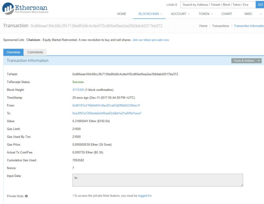
Рис. 21. Etherscan.io
